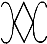
Damıtıcı
